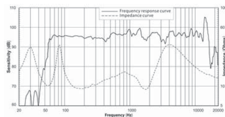
Frekvenční charakteristika
