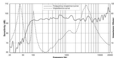
Frekvenční charakteristika
